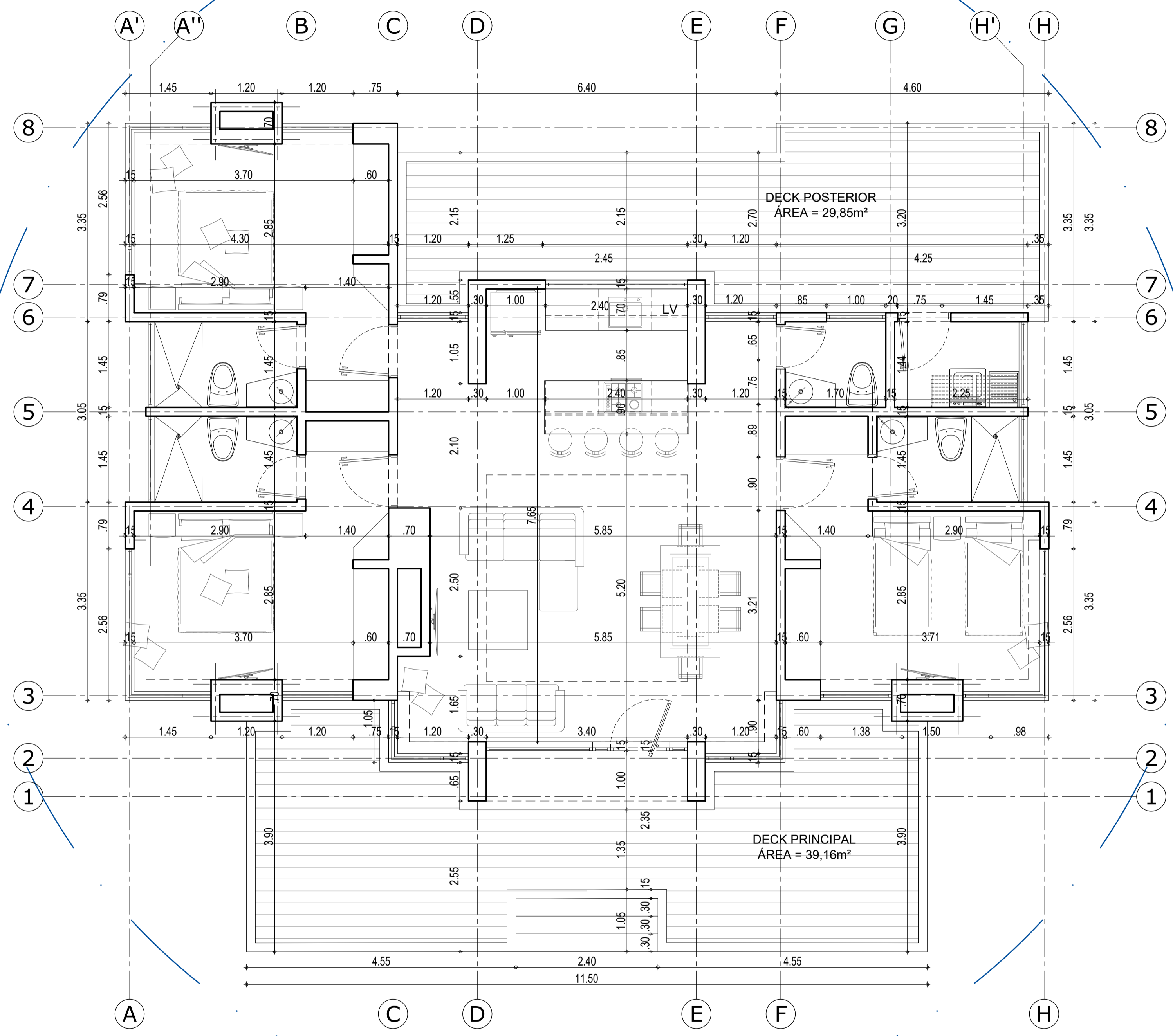
CASA MODELO - 3 ALCOBAS 4 BAÑOS Y CUARTO DE ROPAS ÁREA CUBIERTA = 127,45m 2
